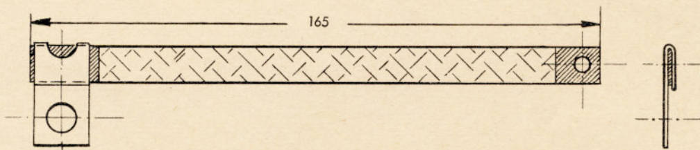
Abb. 3 Masseband kpl. Bestell-Nr. 281 Z 491 Maßstab 1:1,5
