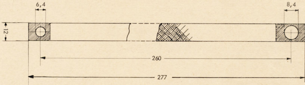
Abb. 2 Masseband kpl. Bestell-Nr. Z400-25 Maßstab 1:1,5
