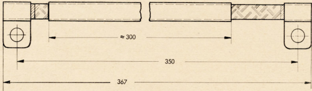
Abb. 1 Masseband kpl. Bestell-Nr. 282 Z 440 Maßstab 1:1,5
