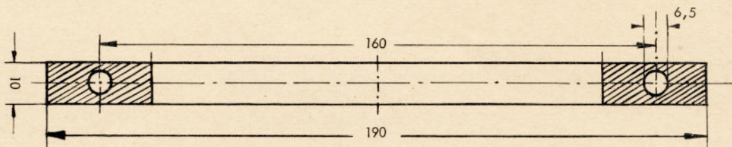
Abb. 4 Masseband kpl. Bestell-Nr. 281 Z 407 a Maßstab 1:1,5
